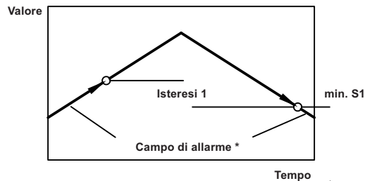
Regolazione min. S1 fig. 8
