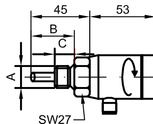
Dimensiones fig. 4
