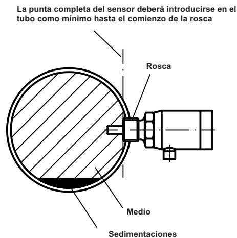
Montaje lateral fig. 2
